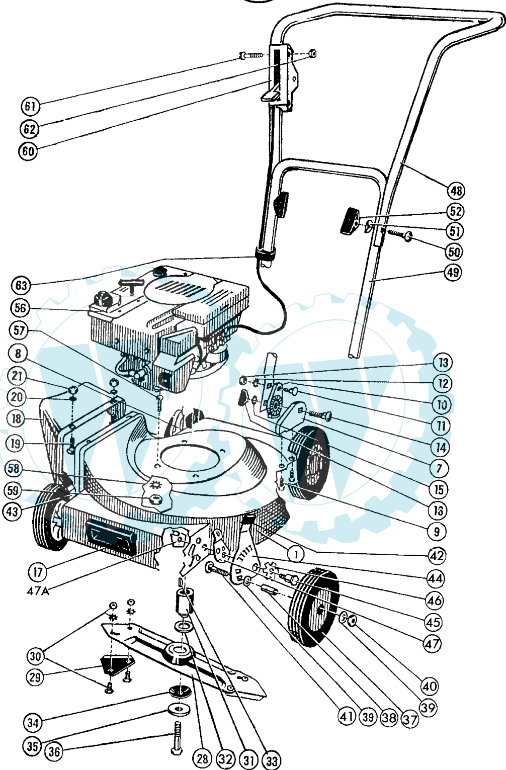
Roto - FOX 46 Typ 1132-01
